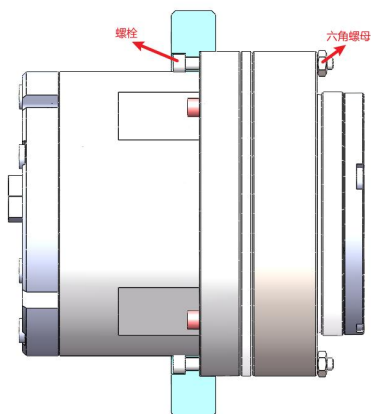
图 18-8 电机外壳固定端锁付模组正确方式
