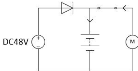
图 8-8 蓄电池充电
