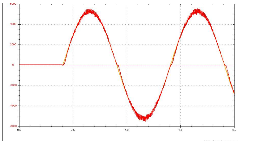
图 15-6 速度环正弦波激励波形
