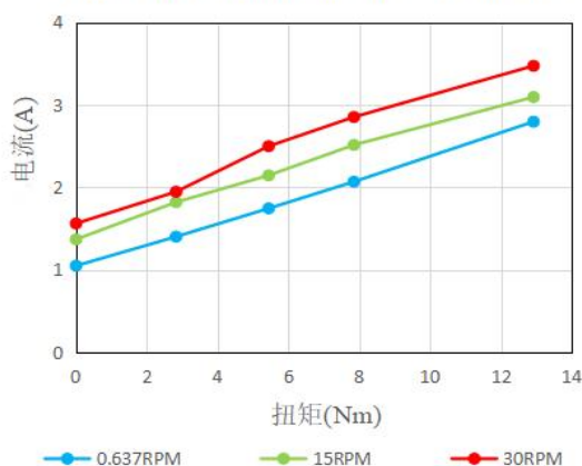
eRob70H100I 电机电流-输出扭矩-转速曲线
