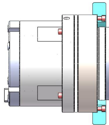
图 18-9 交叉滚子轴承端锁付模组正确方式
