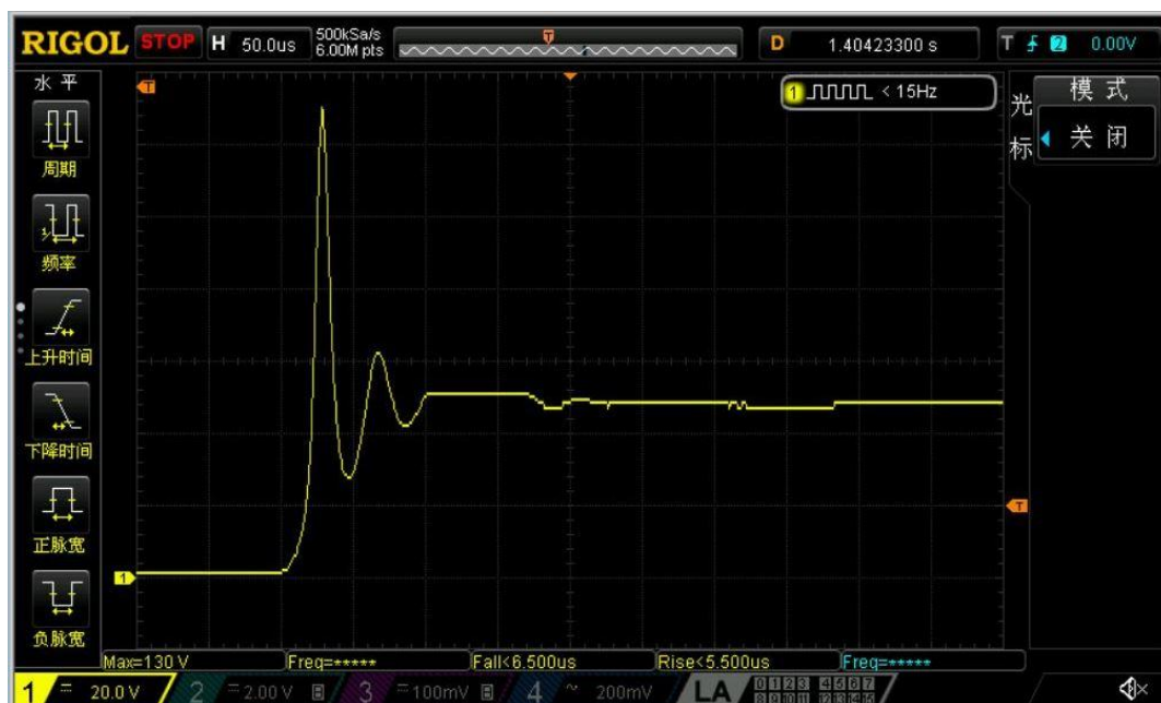
图 3-1 关节异常供电的输入电压波形 (Max=130V>60V)
