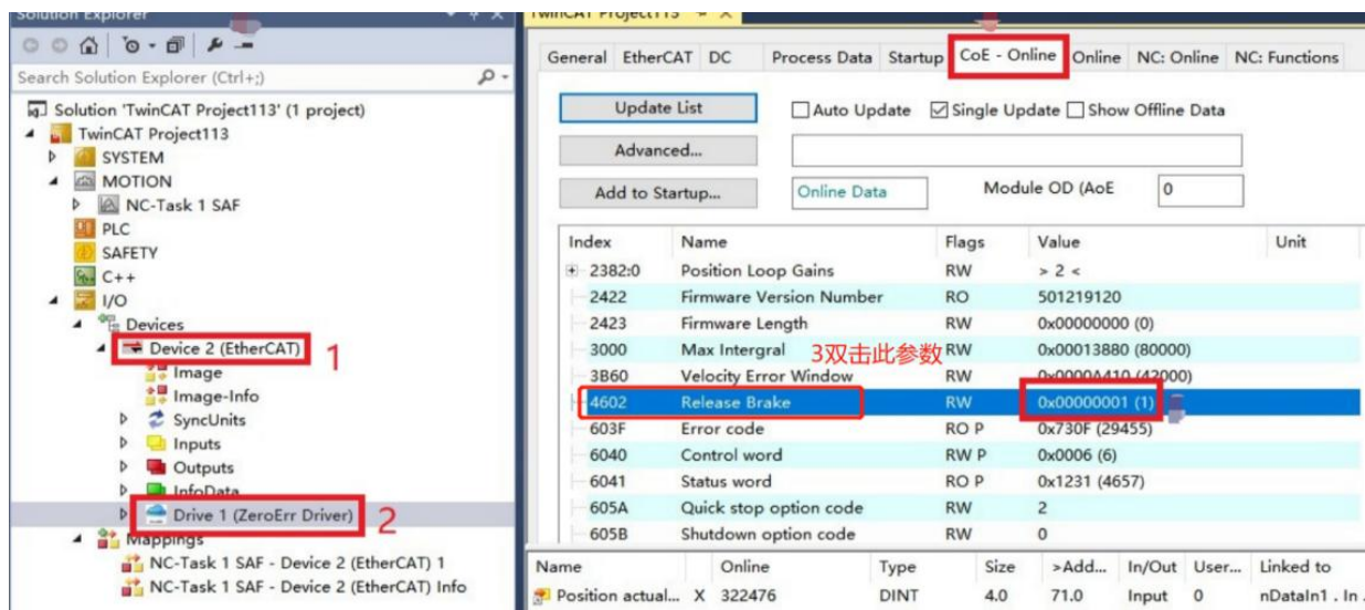
图 7-4 TwinCAT 操作释放刹车
