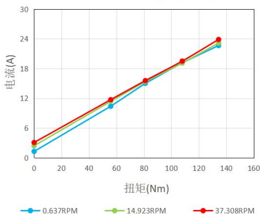
eRob142H120I电机电流-输出扭矩-转速曲线
