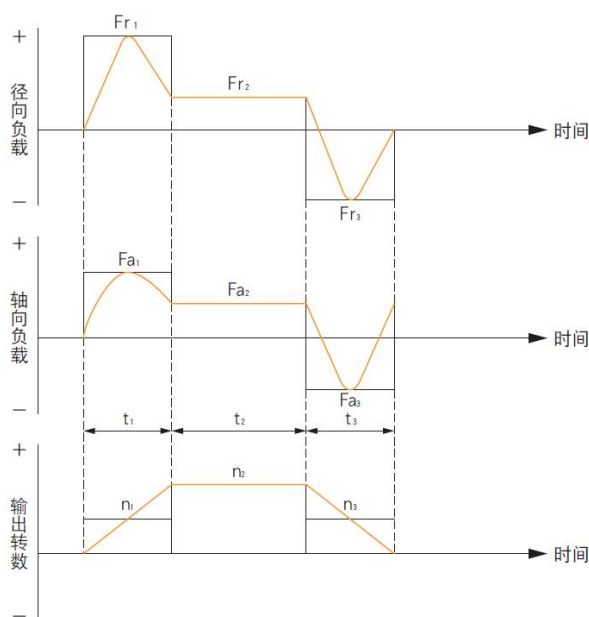
图 17-2 负载模式图
